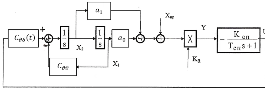
Рис. 1. Структурная схема адаптивной системы управления неустойчивым объектом управления
