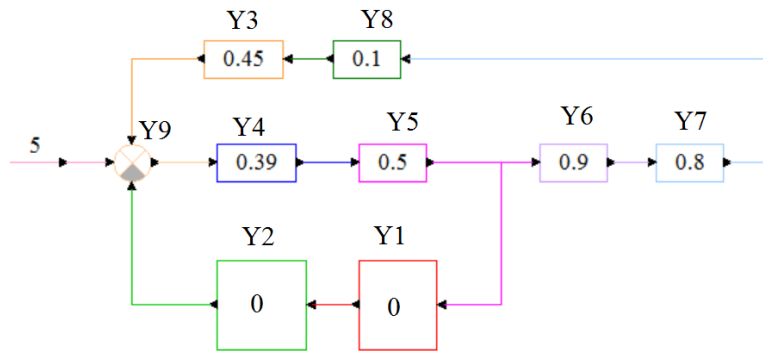
Рис. 20. Структурная схема системы в начальный момент времени Расчет значений выходных сигналов в начальный момент времени осуществляется в продукте MathCAD (рис. 21):
